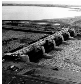
Das Eidersperrwerk ist eines der größten Küstenschutzbauwerke Europas Foto: WSA Tönning
